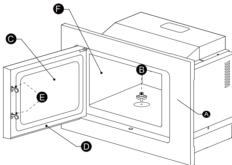
Поворотний вал
